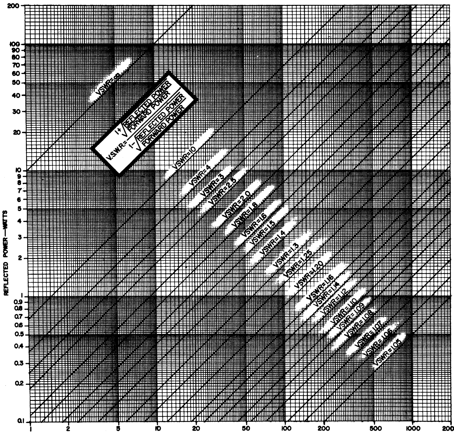
FIG. 4 V.S.W.R. CHART
